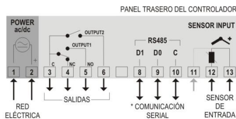
Fig. 1 - Conexiones mostradas en la etiqueta del controlador
