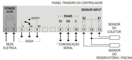
Fig. 1 – Conexões mostradas na etiqueta do controlador
